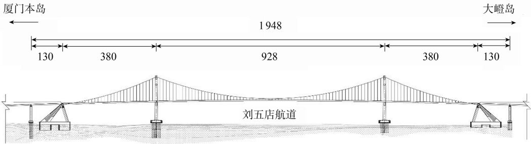
图 1 刘五店航道桥结构示意图(单位:m) Fig. 1 Schematic diagram of Liuwudian Navigation Channel Bridge(unit:m)
