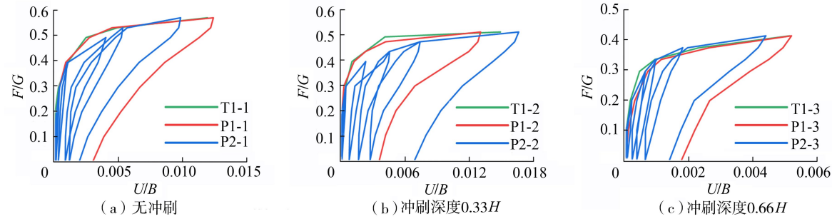
图 4 不同工况下 3 种加载方式锚碇散索鞍处的荷载-位移曲线
