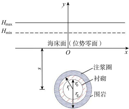
图 1 隧道渗流场简化计算模型
