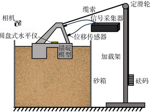
图 3 试验装置示意图 Fig.3 Schematic diagram of the experimental setup
