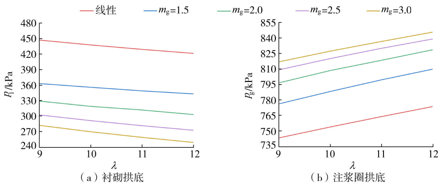
图 11 厚度比对衬砌与注浆圈拱底孔隙水压力的影响
