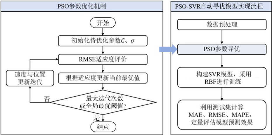
图 2 PSO-SVR 自动寻优模型构建流程
