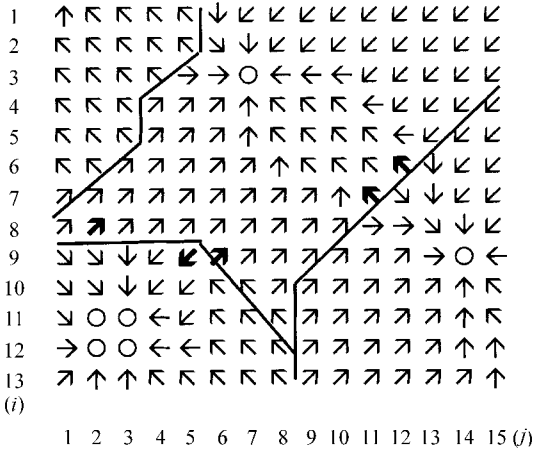
图4 研究区域网格方向示意图
