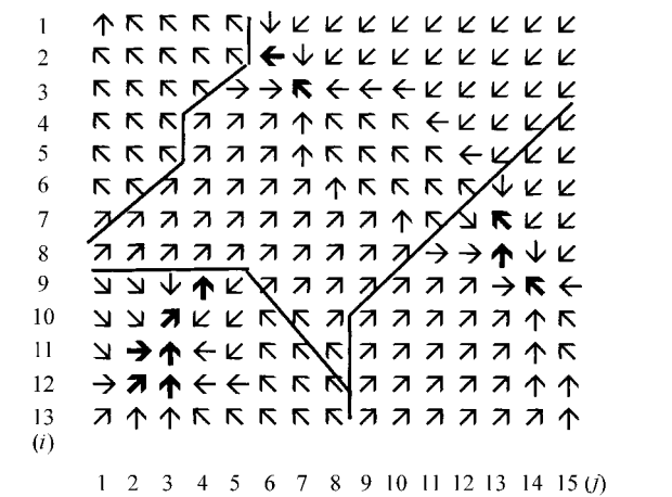
图 6 网格方向示意图
