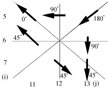
图3 研究区域中 Z (6,12)的方向权重法示意图 Fig.3 An example of MDWM for pixel Z (6,12)
