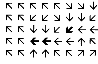
(d) 黑体箭头为修正过的网格方向,即完整的MDWM确定的平地网格方向
