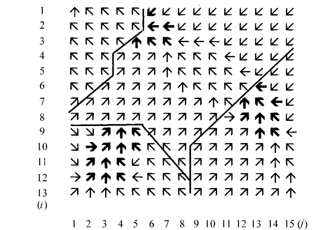
图 7 网格方向示意图
