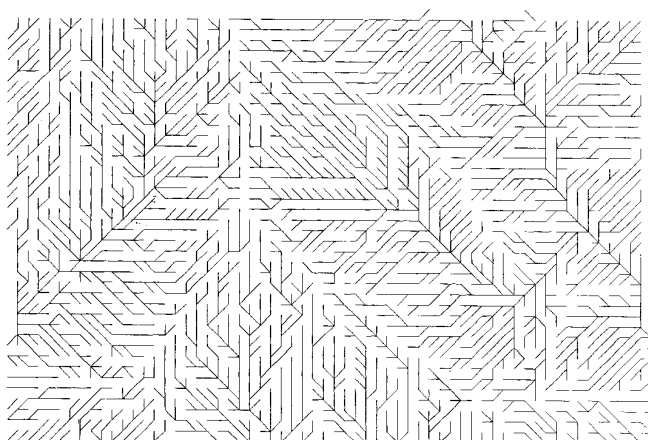
图 10 流域 D 上由 30\text{ m} \times 30\text{ m} 的 DEM 用 ARC/INFO 导出的部分流水网(所示区域同图 8)
