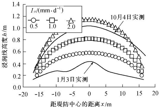
图 5 江户川堤防浸润线的实测值和计算值
