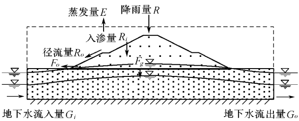
注： F_i —向地基内的流入量； F_o —堤脚的流出量
