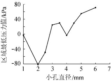
图 5 不同小孔直径时区域最低压力分布曲线
