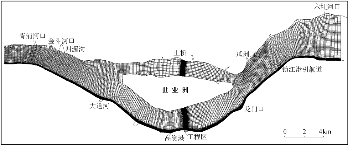
图 2 局部模型计算网格
