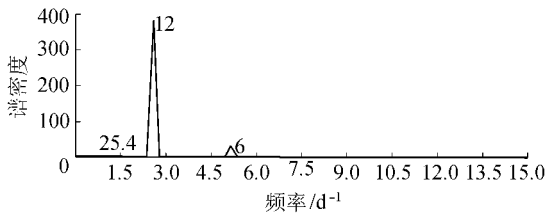
图 5 月均海表温度异常的功率谱分析
