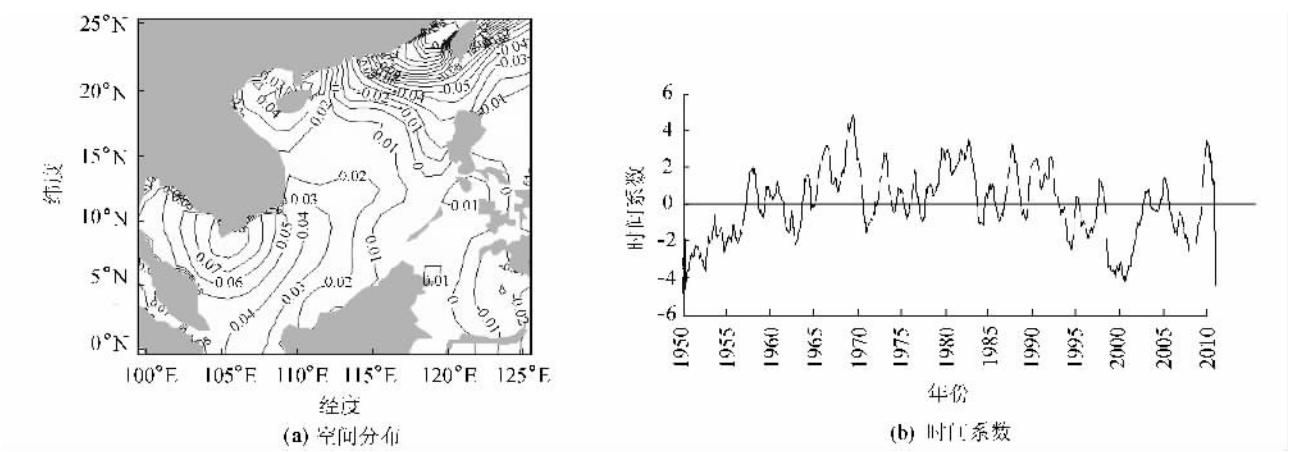
图 8 南海海表温度异常场 EOF 分解第 2 模态的空间分布及其时间系数
