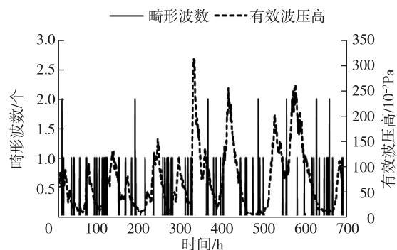
图1 Anmado 测站畸形波个数与有效波压高的关系
