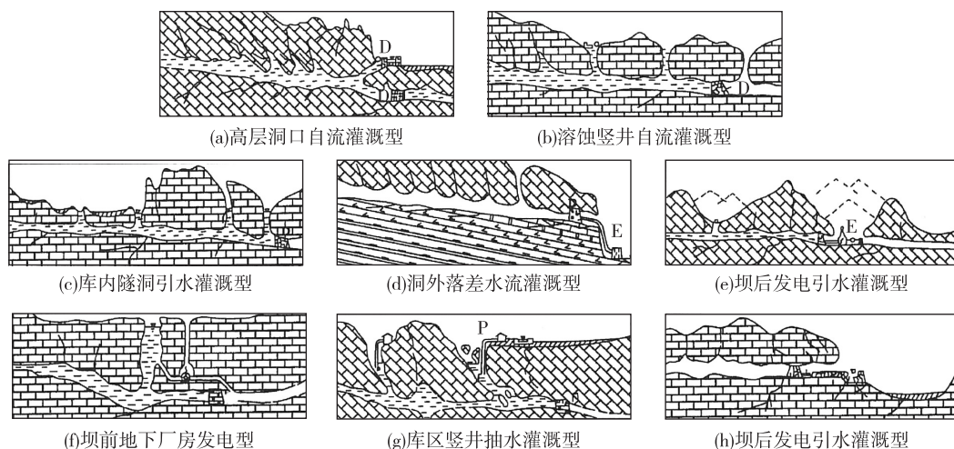
图9 封闭地下坝型地下水库示例
