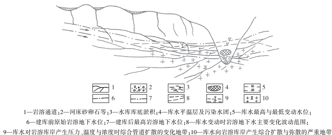
图8 库水对岩溶地下水产生污染分析示意图
