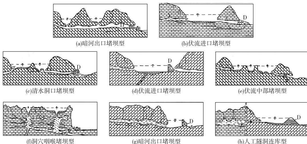
图 11 地表与地下相连水库示例
