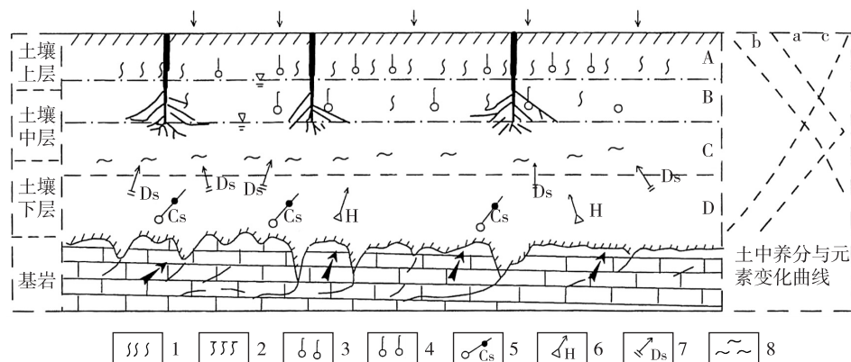
1—第一淋滤作用;2—第二淋滤作用;3—第一蒸发作用;4—第二蒸发作用;5—土壤中浓度扩散作用(可逆); 6—土壤中热力扩散作用(可逆);7—动力扩散作用;8—植物根系吸收作用; A—上部渗透淋滤带;B—淋滤-蒸发带(地下水位变动带);C—土壤养分富集带;D—基岩-土层活跃作用带; 元素变化曲线有三种:a型—Ti、Ni、Zn、Ca、Pb、Hg、As、Bi;b型—Co、Mn;c型—Cr
