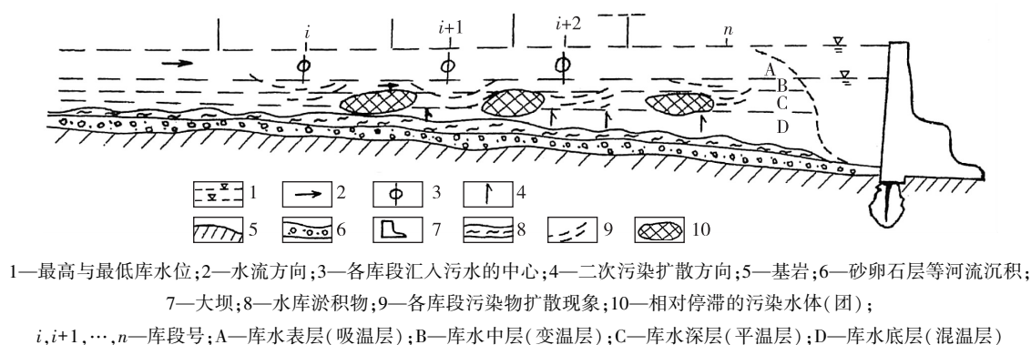
图7 水库污染状况理论分析示意图
