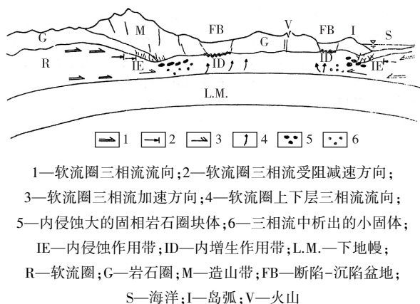
图2 软流圈内侵蚀与内增生作用理论分析
