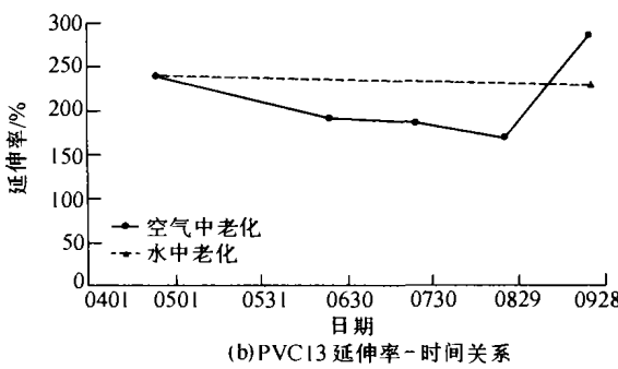
图 1 PVC13 土工膜老化性能
