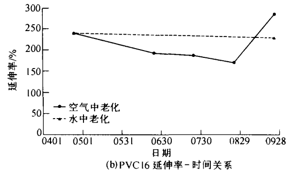
图 2 PVC16 土工膜老化性能
