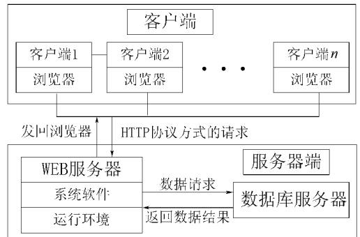
图 2 B/S 模式的网络结构
