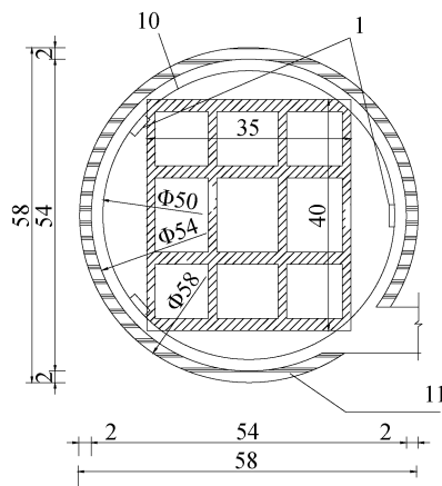
(b) 俯视图
