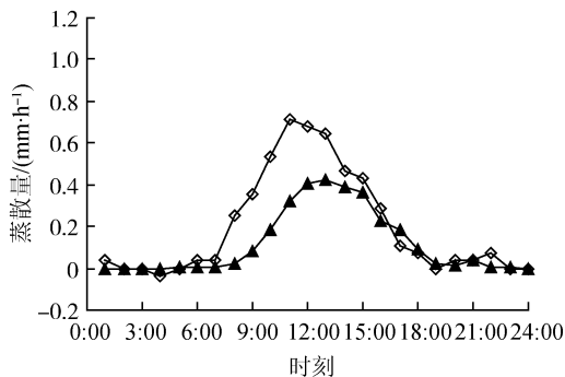
(d) 拔节孕穗期(8月29日)
