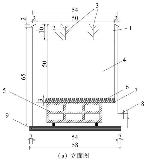
(a) 立面图
