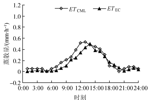
(a) 分蘖前期(7月10日)
