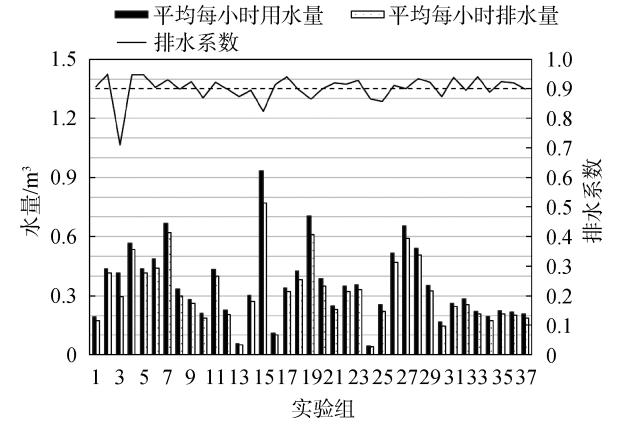
图 1 办公楼排水系数测定
