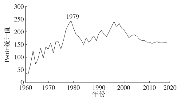
图3 海河流域年降水量突变分析
