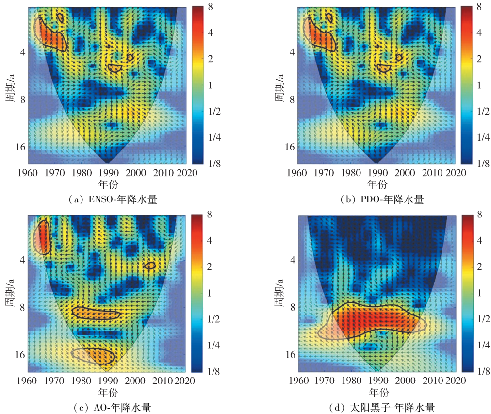
图 6 海河流域年降水量与 ENSO、PDO、AO 以及太阳黑子的交叉小波功率谱
